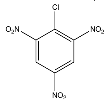
2-chloro-1,3,5-trinitrobenzene
